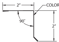
AAF2210
